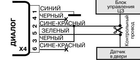
Рис. 11. Схема подключения к центральному замку, которому для отпирания требуется отрицательный импульс, а для запирания - разъединение проводов
