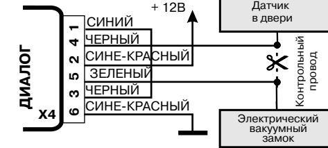
Рис. 10. Схема подключения к вакуумному центральному замку
